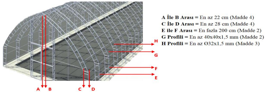
Şekil 3b - Portatif Çadır Ağıl İskelet Şeması
