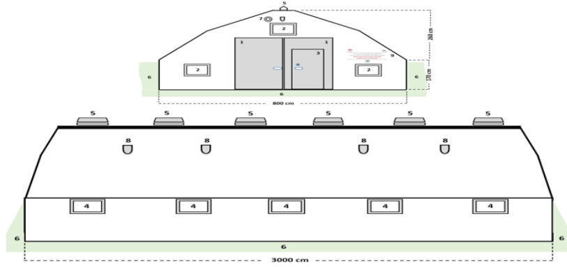
Şekil 2a- Portatif Çadır Ağıl (8x30)
