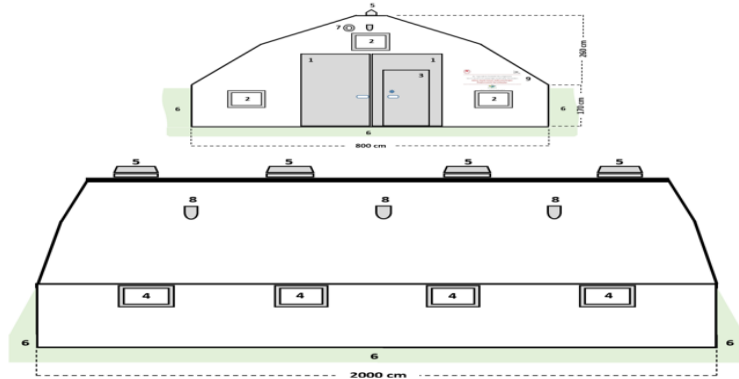
Şekil 2b- Portatif Çadır Ağıl (8x20)
